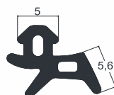
Прокладка окна из ПВХ черного цвета
