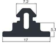
HM01 CEPHE FITİLİ Aluminium Face Gasket
