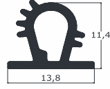
ALD04 CAM FITİLİ Glass Gasket
